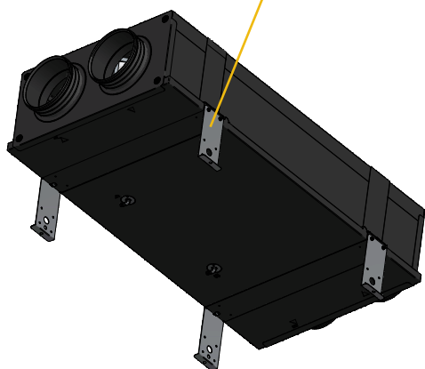
Piedi per installazione a pavimento Feet for floor installation
