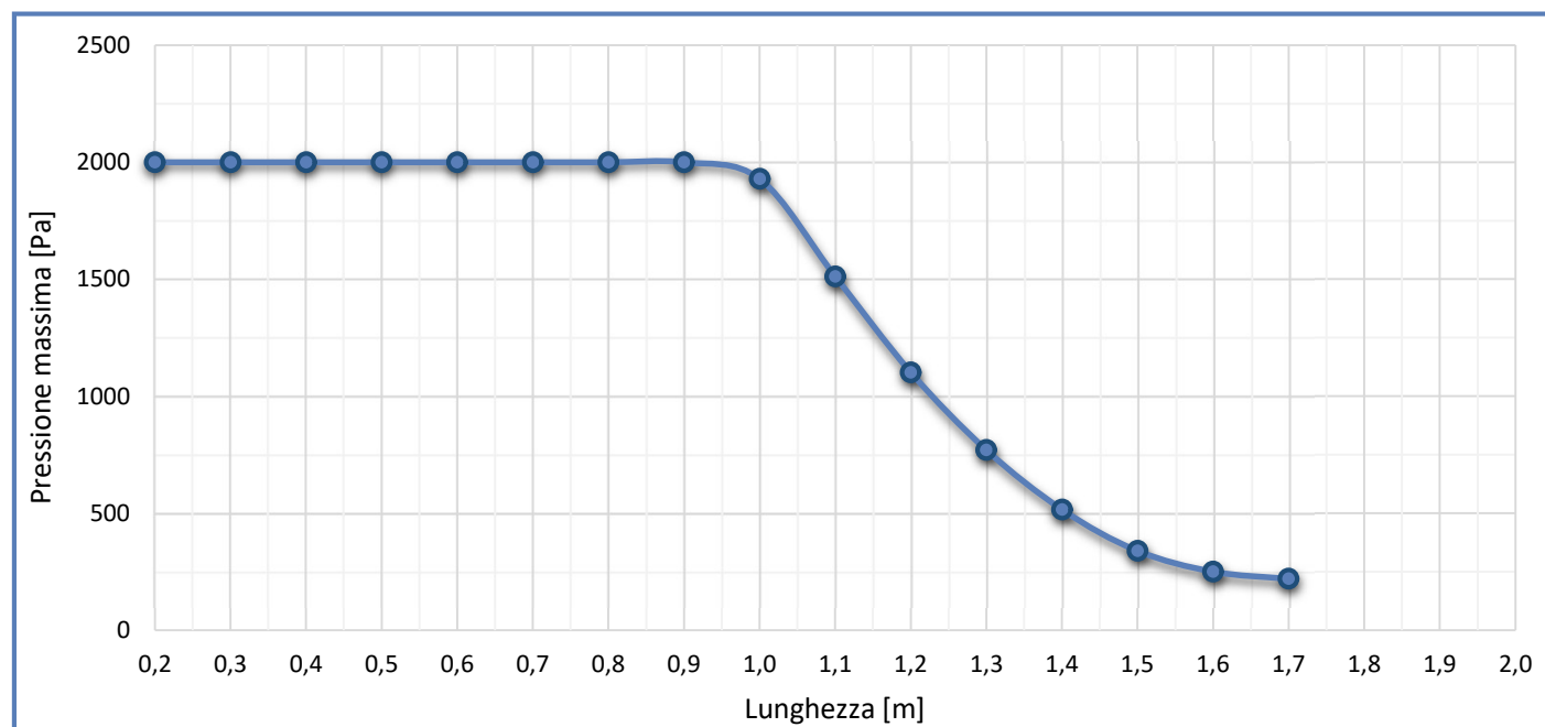
Grafico Pressione Massima Ammissibile DLT 100 ZA
