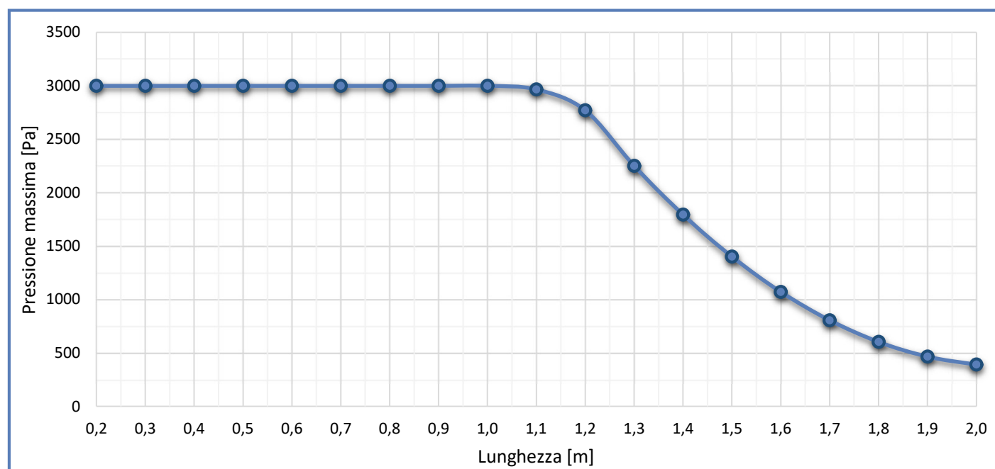
Grafico Pressione Massima Ammissibile DLT 150 X - XX
