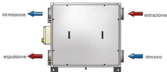
DUO-EC V – VISTA LATERALE Configurazione specchiata
