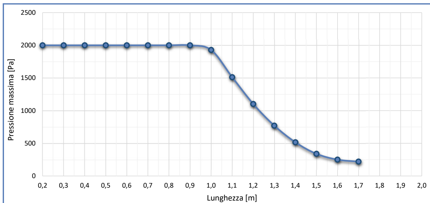
Grafico Pressione Massima Ammissibile LDT-T 100 ZA
