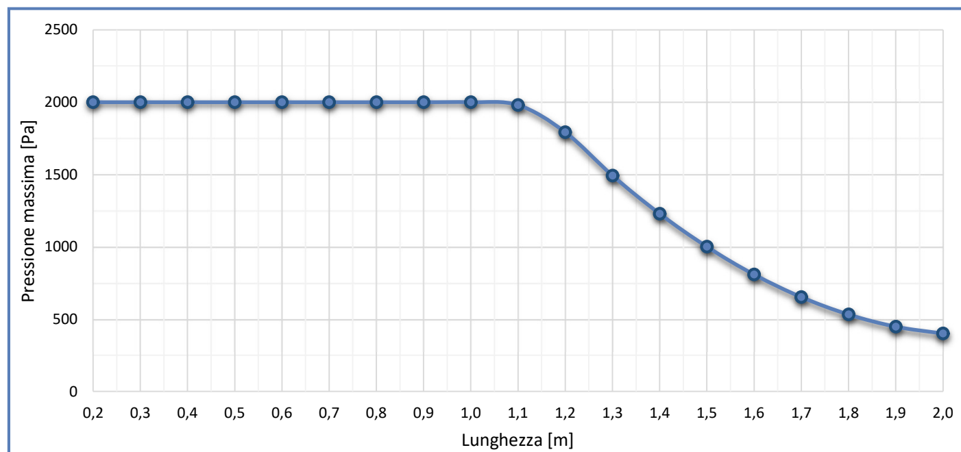
Grafico Pressione Massima Ammissibile LDT-T 150 A
