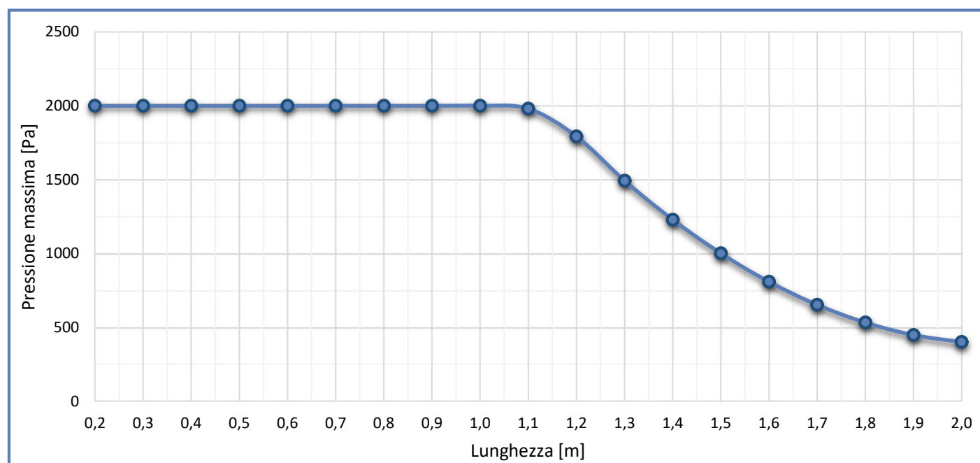
Grafico Pressione Massima Ammissibile LDT-T 150 ZA
