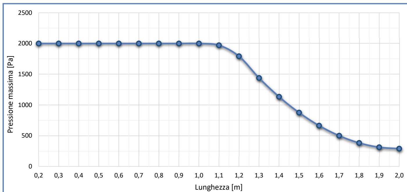
Grafico Pressione Massima Ammissibile LDT-T 200 X-XX
