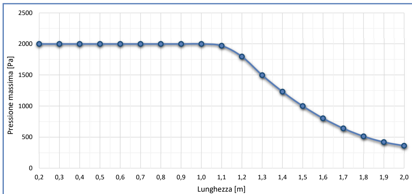
Grafico Pressione Massima Ammissibile LDT-T 200 ZA
