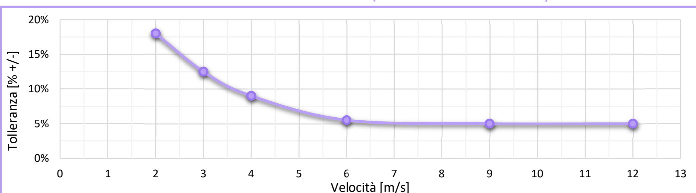
Grafico Percentuale Incertezza Sonda (in condizione di installazione)
