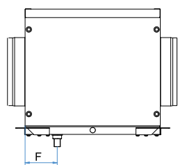
DIMENSIONI (mm)
