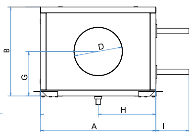
DIMENSIONI (mm)
