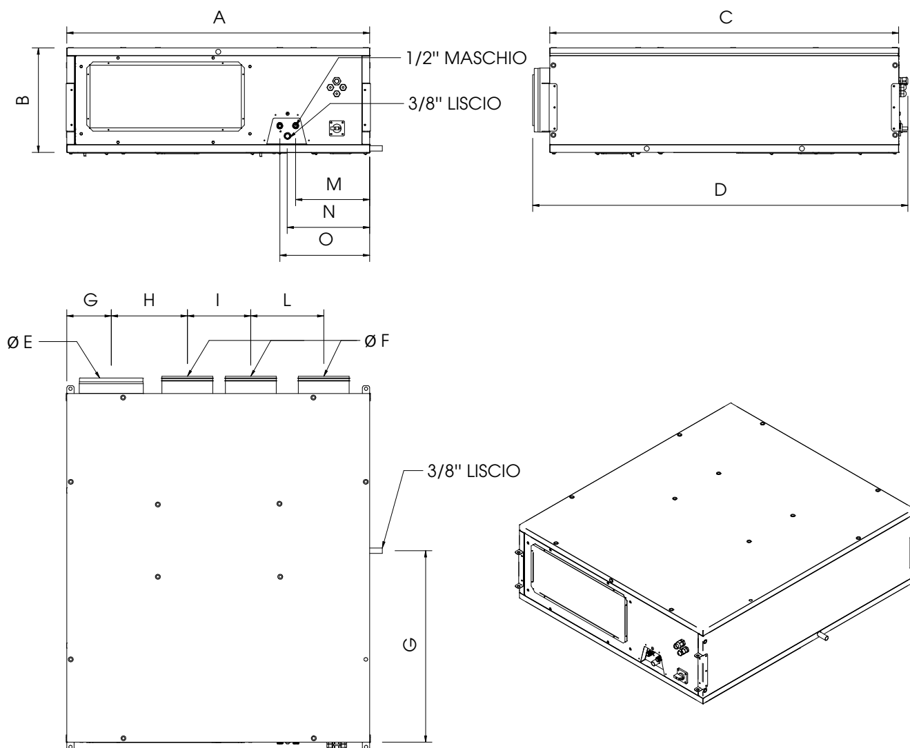
DIMENSIONI [mm] e PESO [kg]
